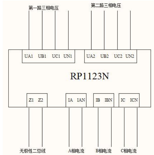
图 传感器接线示意图
